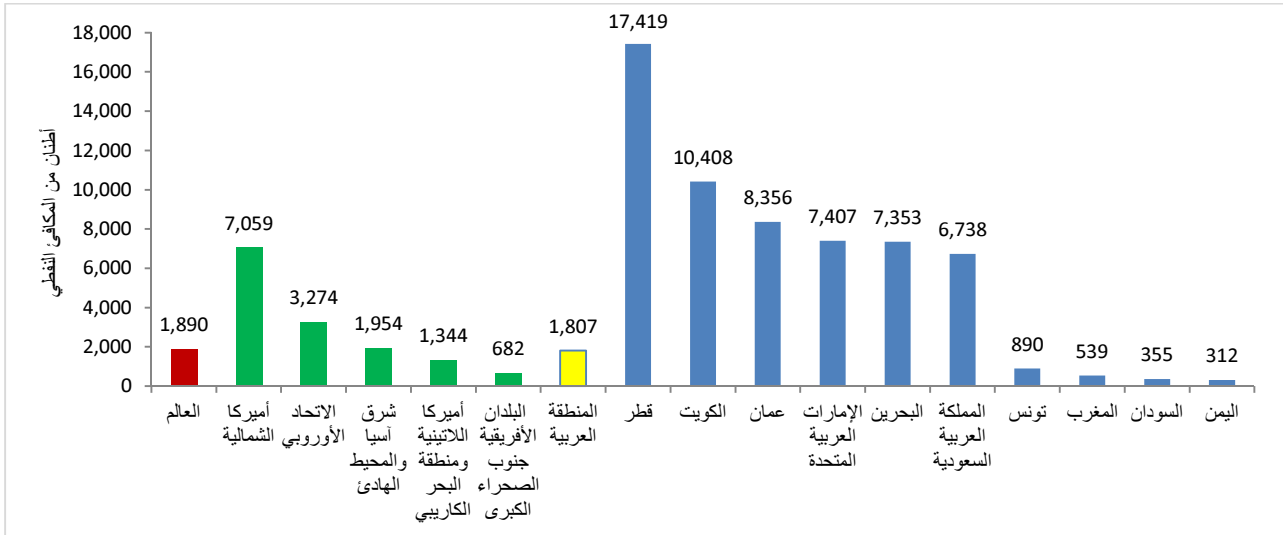
الشكل: استهلاك الطاقة للفرد الواحد – الدول العربية وبقية العالم (٢٠١١) (كيلوغرام مكافئ نفطي)
